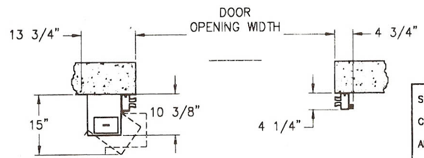
SECTION A-A
